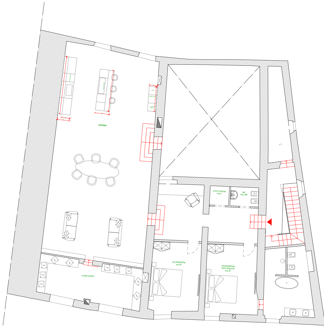
PIANO TERZO – Livello +1
